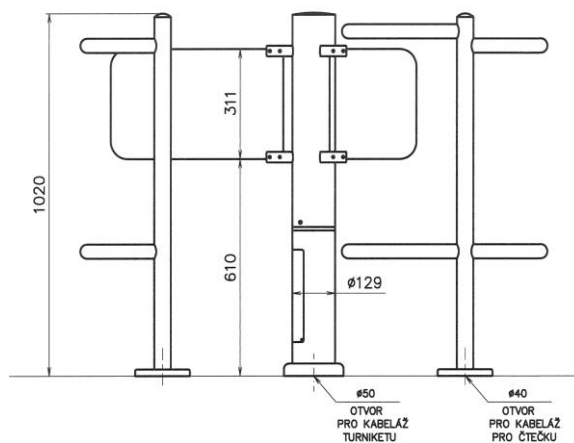
IVRY-TRM1S nákresy
